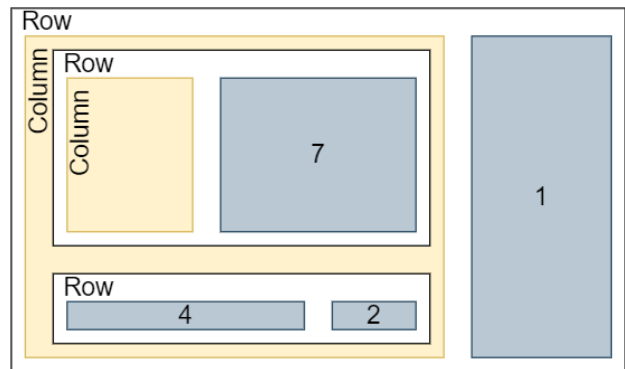
Abbildung 20. Keine der zwei Rows beinhaltet nur einen Chart, weshalb beide gesetzt werden
